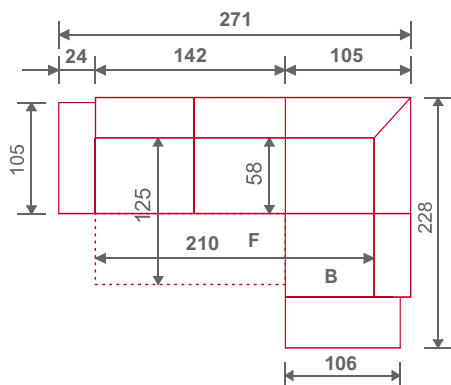
S01 (26F*+50+41B*)
